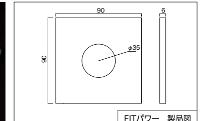
専用スペーサー:亜鉛メッキ
