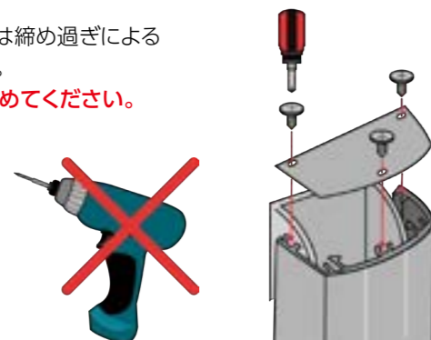
①化粧小口穴合わせ ②ビスで固定
