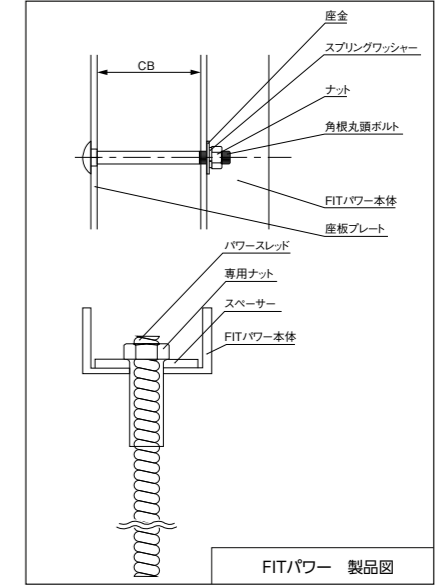
ロックボルトは1柱当たり2セット
